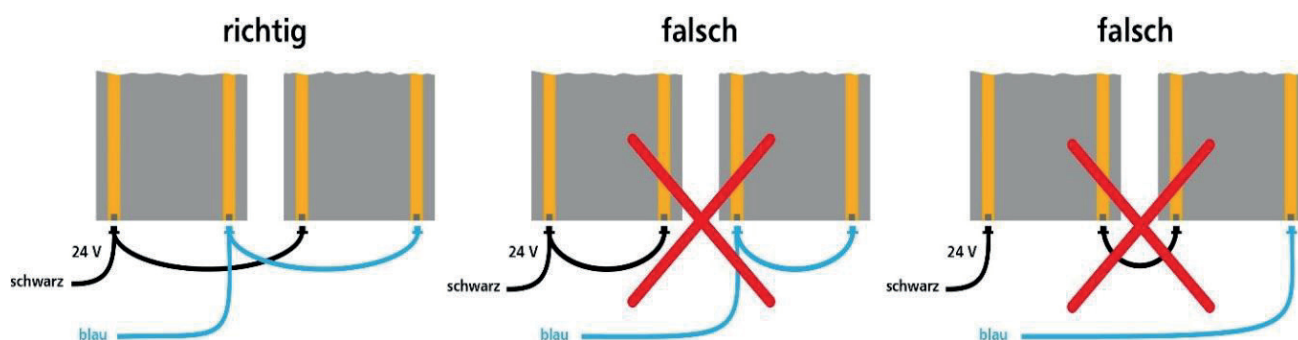
Abbildung 9: Bei einer geteilten thermoheld Trockenbauplatte 36V können die einzelnen Platten (bis maximal 8 Heizfelder bzw. 300 W) durch Wago Klemmen in Unterputzdosen wieder zusammengeschlossen werden. Hier ist die korrekte und die fehlerhafte Verbindung der Heizstränge dargestellt.
