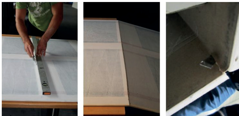
Abbildung 7: Zum Teilen der thermoheld Trockenbauplatte 36V erst sauber anreißen, dann Platte brechen und zum Schluss rückseitigen Karton durchtrennen
