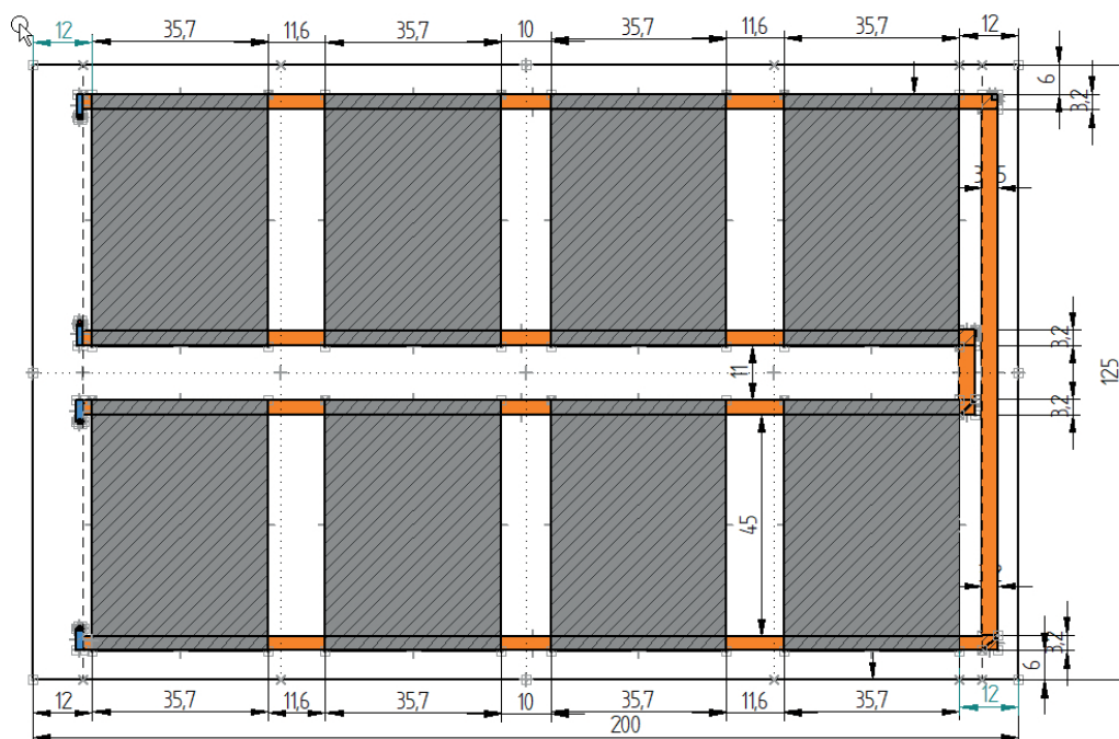
Abbildung 1: Technische Zeichnung thermoheld Trockenbauplatte 36V, Vorderseite, Bemaßung in cm
